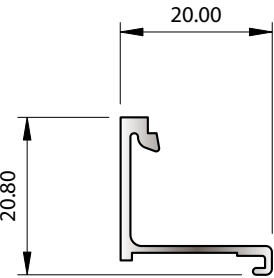
SECTION No. 34245 0.155 kg/m P = 95.43
